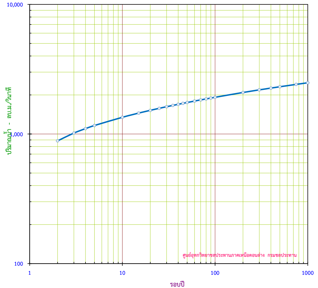
กราฟแสดง ปริมาณน้ำสูงสุดรายปี ขนาดรอบปีต่างๆ สถานี P.12C อ.สามเงา จ.ตาก
